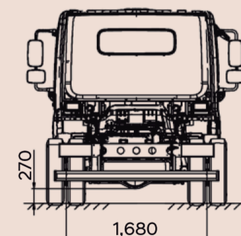
DIMENSIONES FRONTAL Y POSTERIOR
